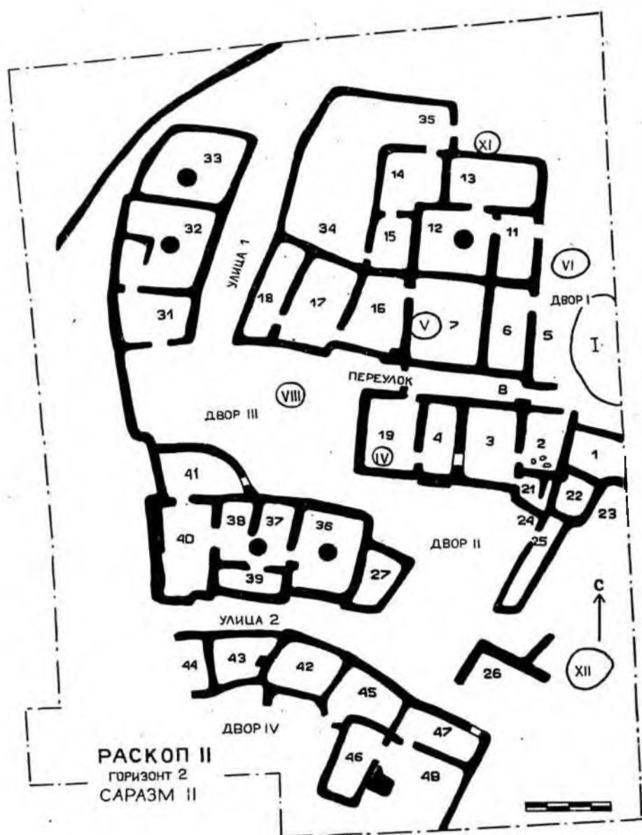
Рис. 8. Раскоп II. План строений горизонта 2. Саразм II.
