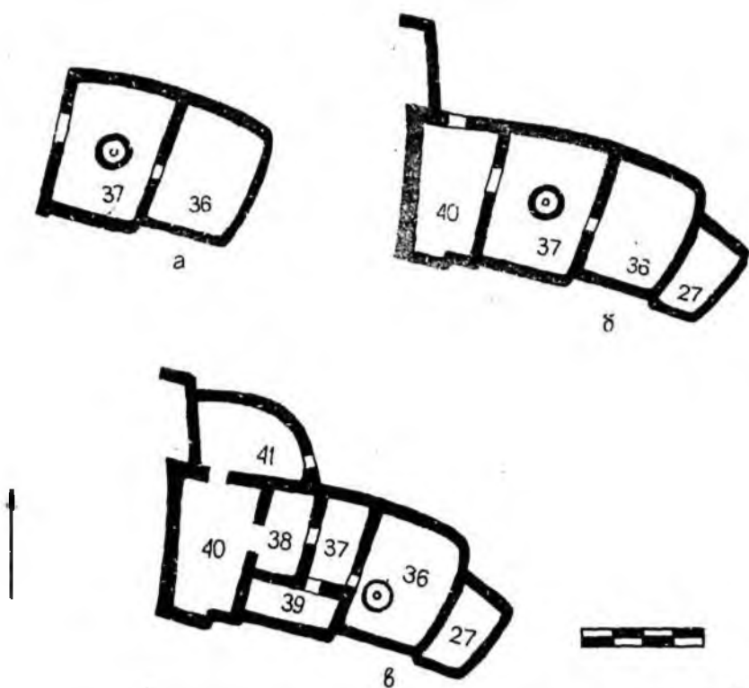
Рис. 16. Раскоп II. План строения шестого жилого комплекса: а, б, в - этапы застройки
