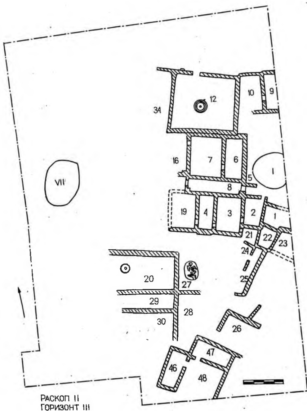
Рис. 18. Раскоп II. План строений горизонта 3. Саразм Ш.
