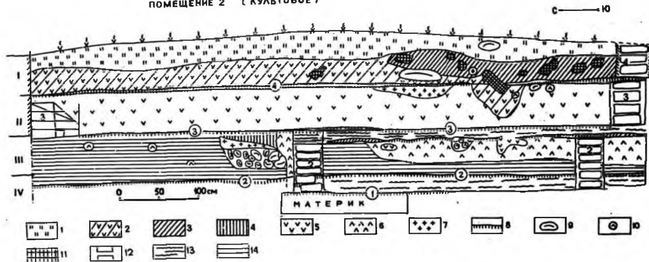
Рис. 66. Раскоп IV. Археологический разрез. Пом. 2: 4-этап В; 3-этап В; 2-этап А1; 1-этап А. Условные обозначения: 1-пахотный слой; 2-рыхлый завал; 3-завал красного цвета-горелый; 4-плотная глина; 5-завал с разложившимися кирпичами; 6-серая земля с золой; 7-обгорелая древесина; 8-полы; 9-камень; 10-фрагменты керамики; 11-кирпичи; 12-кладка стен; 13-гумус; 14-плотный утрамбованный завал
